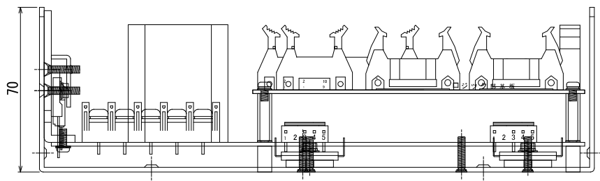
【取付図】 BMC2XH-nn
