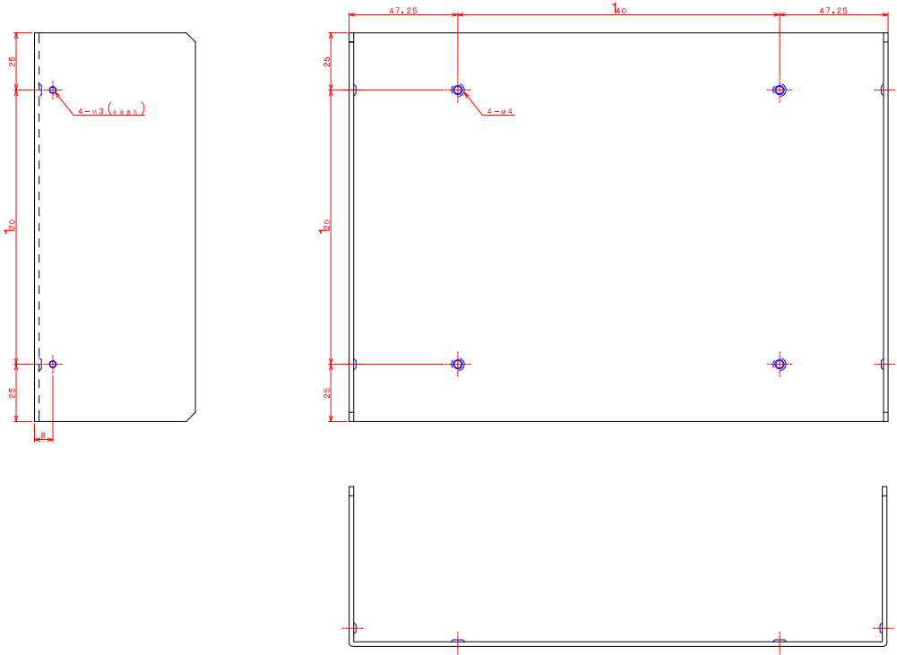
【取付図】 BMC2XH-nn
