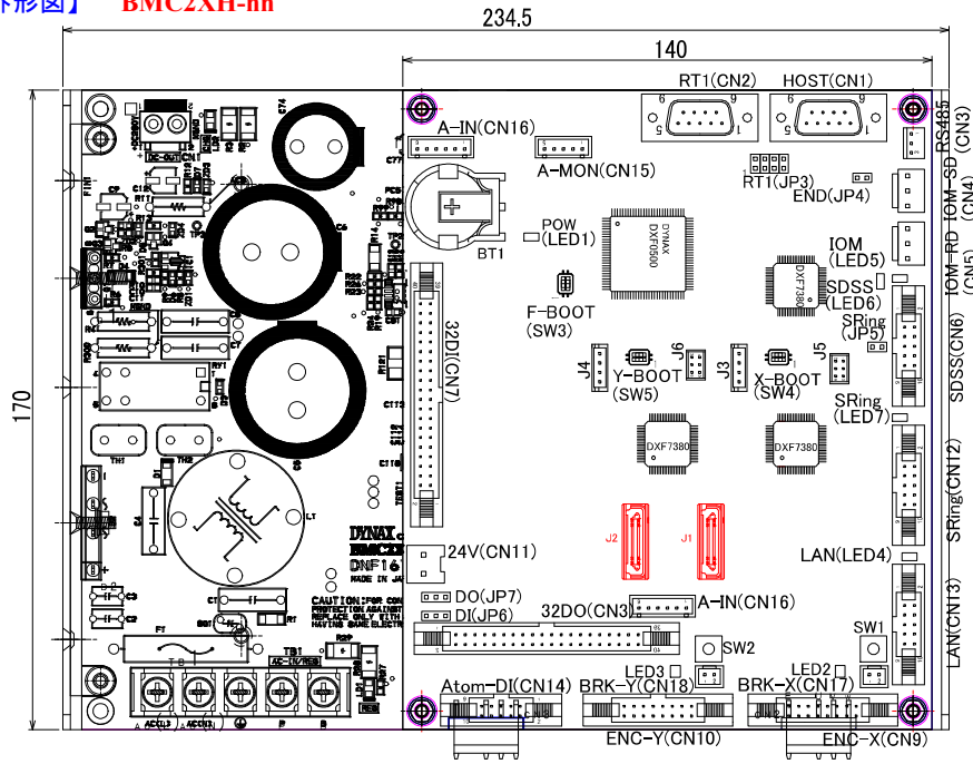
【外形図】 BMC2XH-nn
